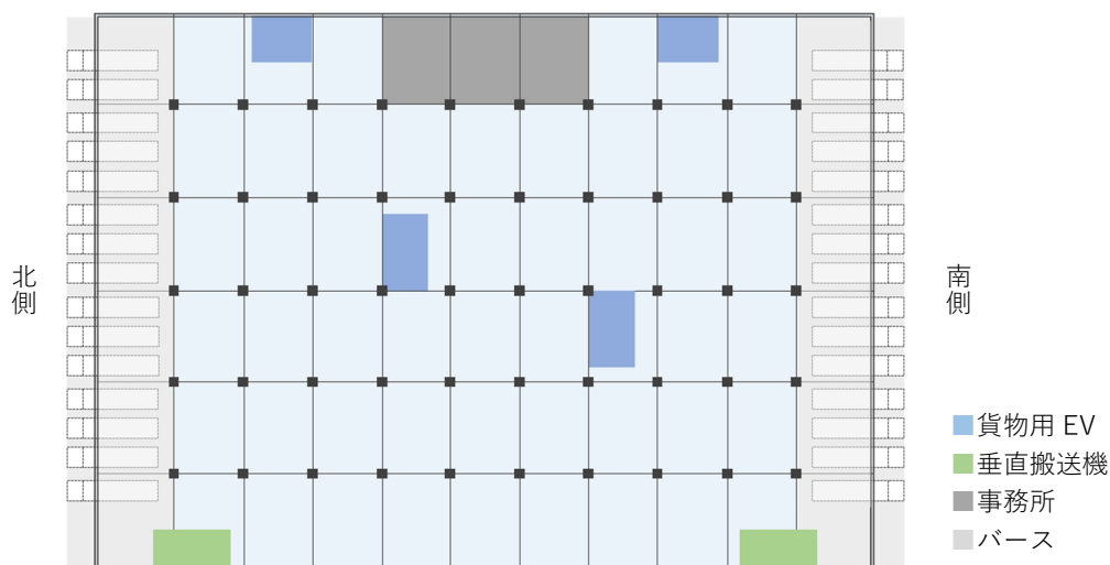
【配置図 (1階)】
